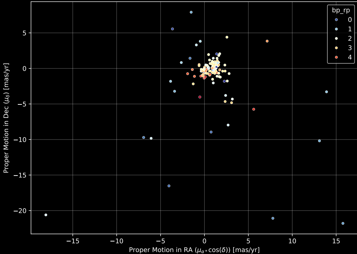
APOGEE DR17 Field: [ORIONNB-RV_btx] Proper Motion Diagram (n= 137)
