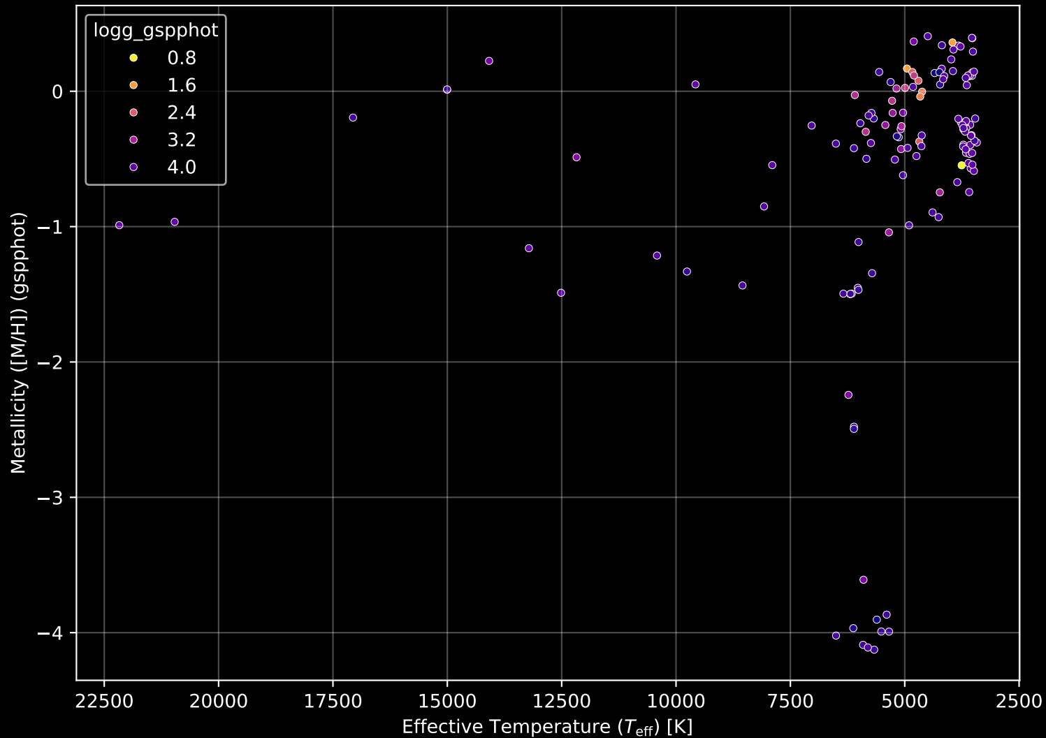
APOGEE DR17 Field: [ORIONB-RV_btx] Stellar Population Parameters (n= 137)
